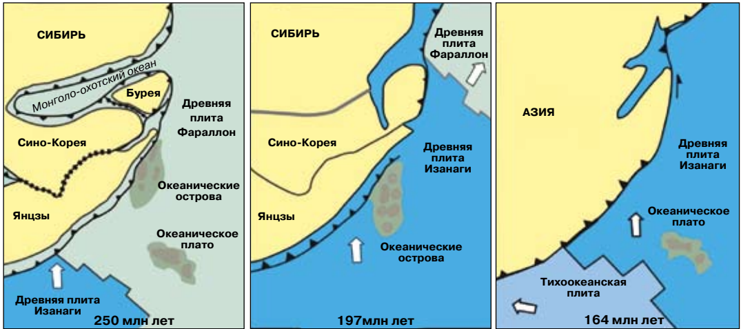
Эволюция Тихого океана в зоне Японской островной дуги 250—164 млн лет назад. Рисунок из книги: Maruyama Sh., Isozaki Yu., Kimura G., Terabayashi M. Paleogeographic maps of the Japanese Islands: Plate tectonic synthesis from 750 Ma to the present. Island Arc 6, 1997. 121—142.
